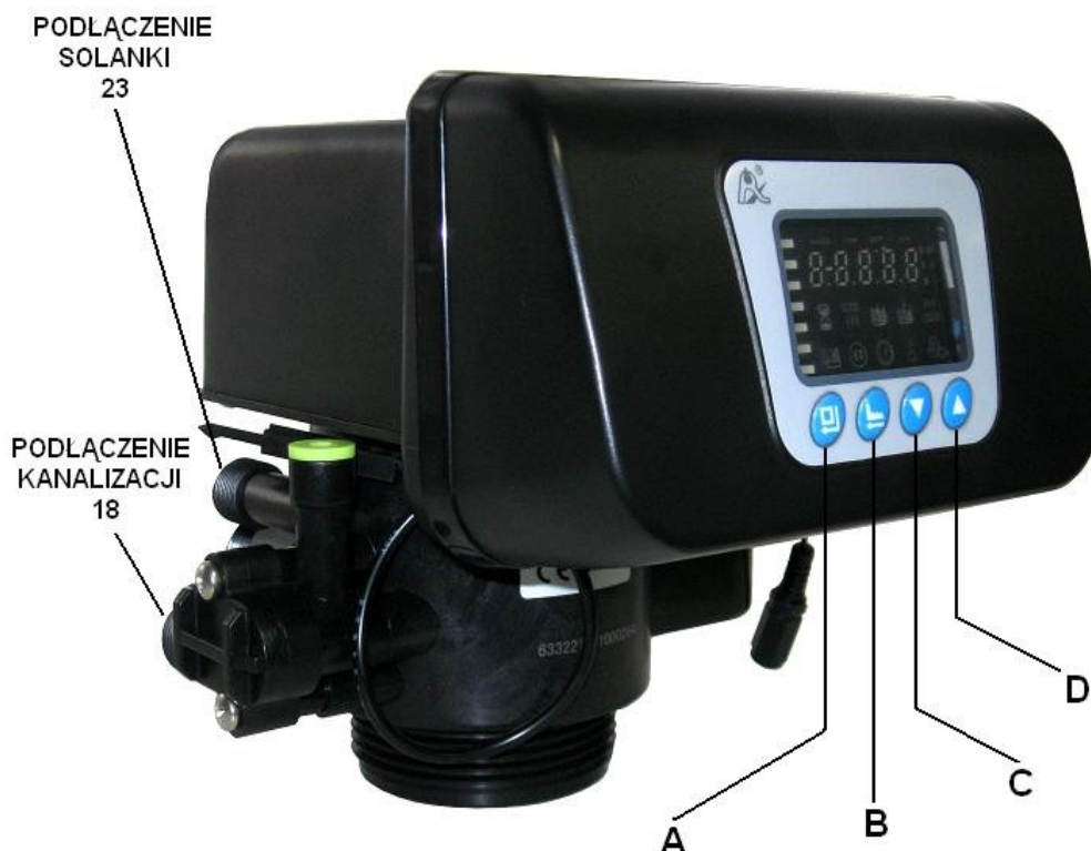
Rys. A. Sterownik RX63C3
